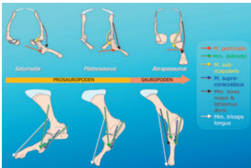
Abb. 4 Beispiel zur Evolution von Schultergürtel und Oberarm der Sauropoden. Oben Ansicht von hinten, unten Ansicht von der Seite. (Erläuterungen siehe Text)
